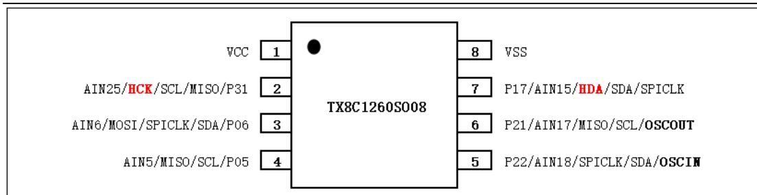
图 5 - TX8C1260S008 (SOP8) 封装图
