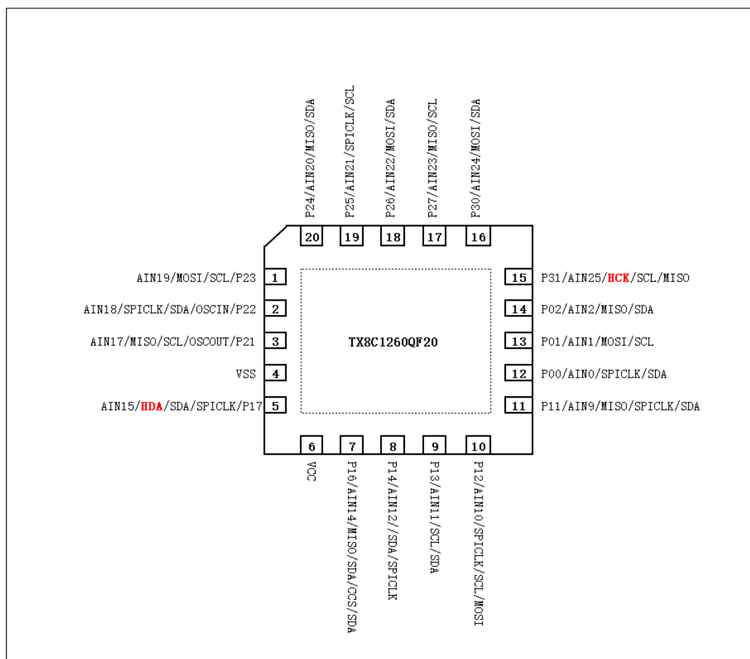
图 2 - TX8C1260QF20 (QFN20) 封装图
