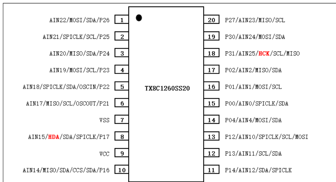
图 4 - TX8C1260SS20 (SSOP20) 封装图
